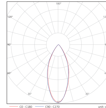
Beam Angle: 45°
