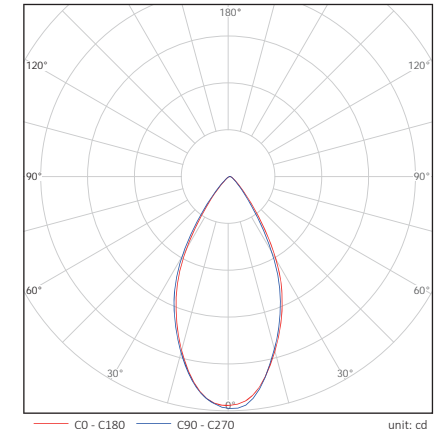
Beam Angle: 60°
